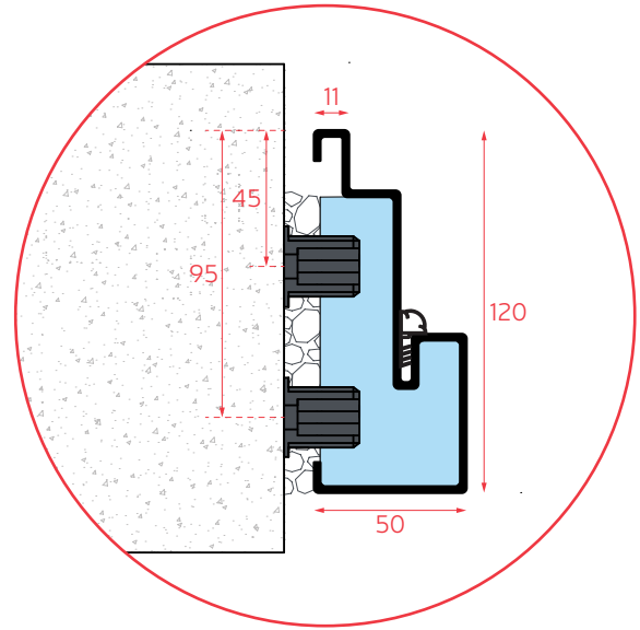
KAMPINĖ STAKTA SU ANGOKRAŠČIŲ APVADAIS
